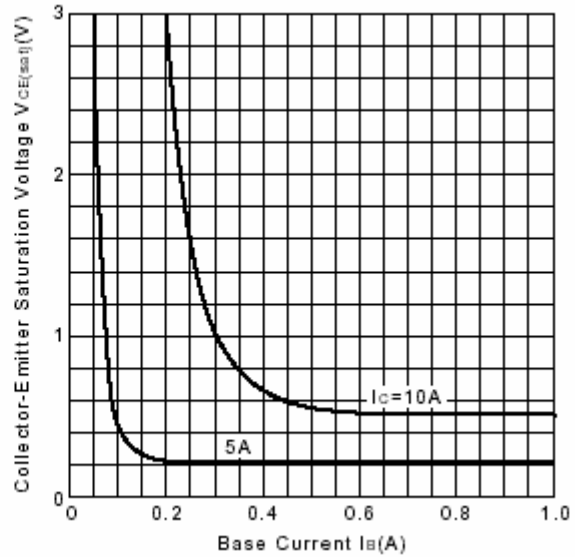
Fig.4 V_{CE(sat)}-I_B
